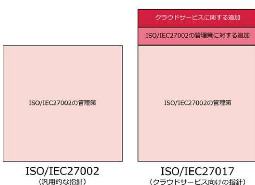
図2. ISO/IEC27002 とISO/IEC27017の体系イメージ
